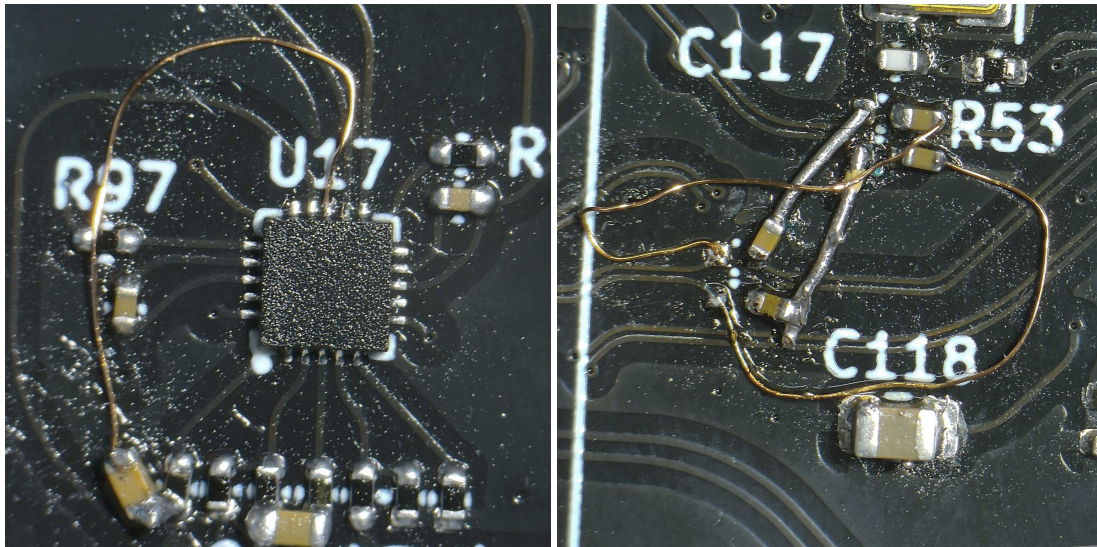
(a) Firul ce leaga unul dintre LDO-uri de un condensator. (b) Repararea liniilor USB prin lipirea unor fire foarte subțiri.
